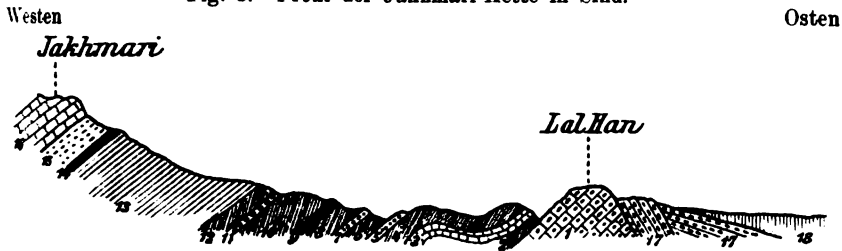
Fig. 3. Profil der Jakhmari-Kette in Sind.
